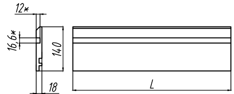
Плинтус рс03_140
