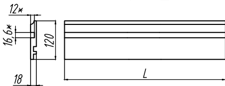
Плинтус рс01_120
