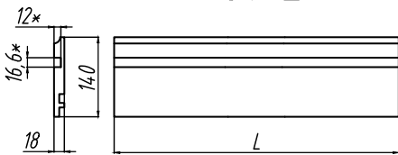
Плинтус рс01_140
