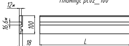
Плинтус рс02_100
