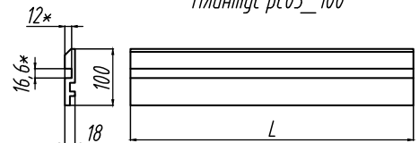
Плинтус рс03_100
