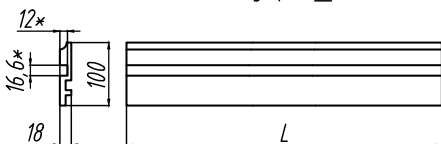
Плинтус рс01_100
