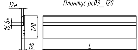
Плинтус рс03_120
