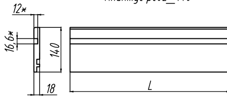
Плинтус рс02_140
